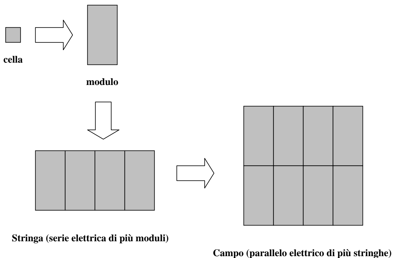
Figura 5: CONFIGURAZIONE DI UN IMPIANTO FOTOVOLTAICO
