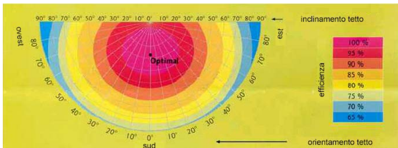
Figura 6: EFFICIENZA DEL GENERATORE IN FUNZIONE DELL'INCLINAZIONE E DELL'ORIENTAMENTO DEL TETTO
