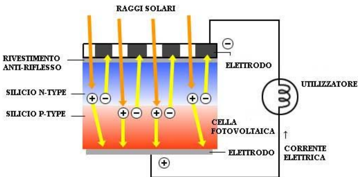
Figura 2: SCHEMA DI FUNZIONAMENTO DI UNA CELLA FOTOVOLTAICA
